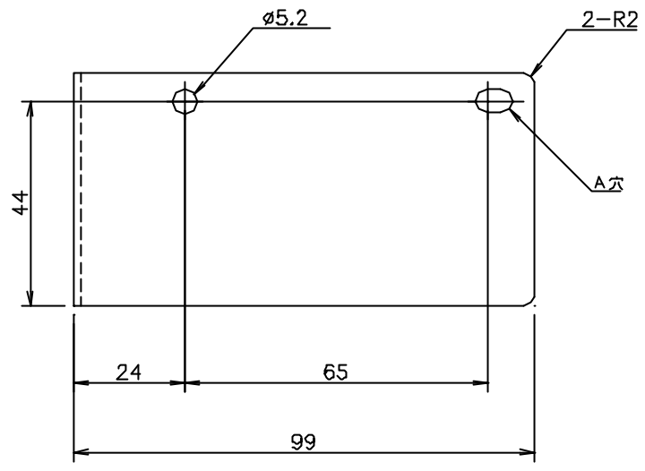
A穴詳細図 (SCALE 2/1)
